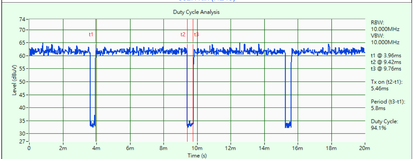
802.11ax (HE80)
