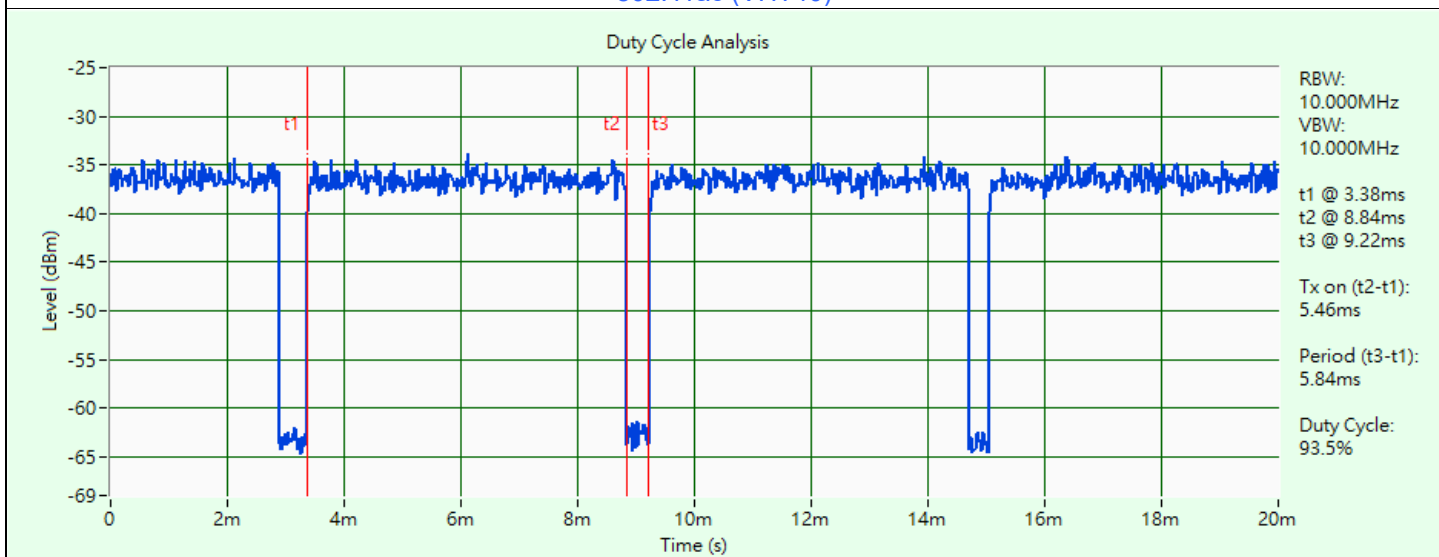
802.11ac (VHT80)
