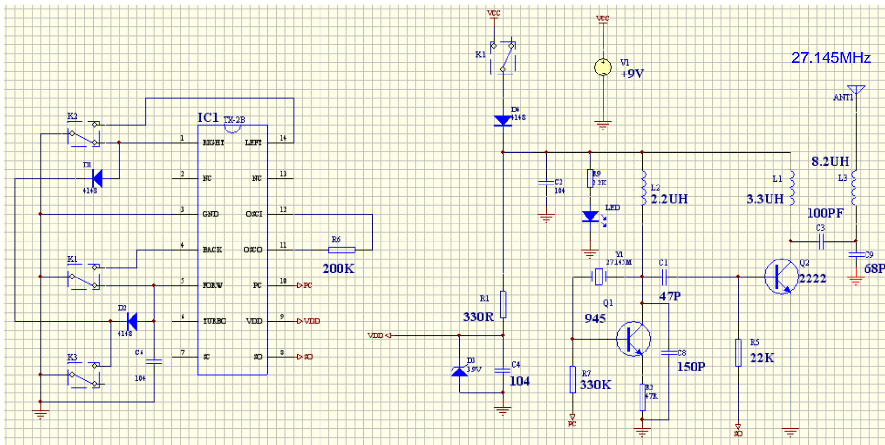
五轮车27M发射线路图
