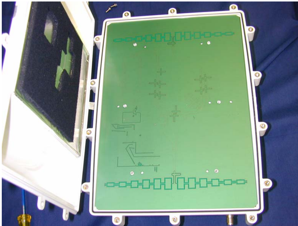
Int. Antenna
