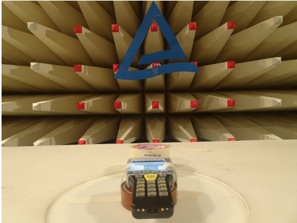
EUT Setup
