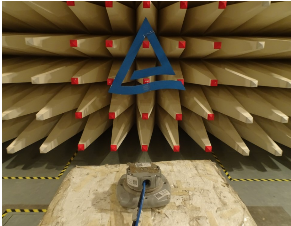
EUT setup
