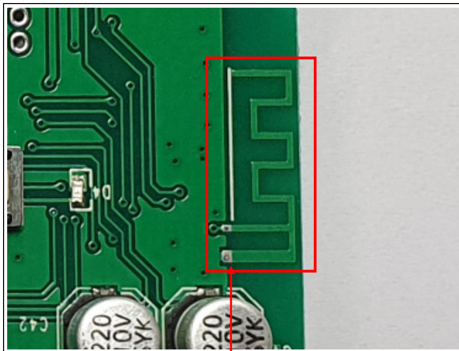
Bluetooth Module
