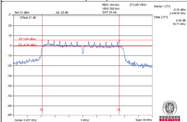
802.11n (HT20) : CH10
