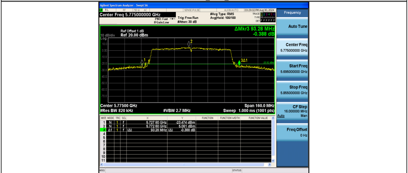
11AC80SISO_Ant1_5775
