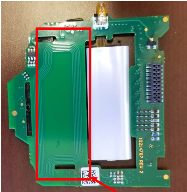
RFID Antenna
