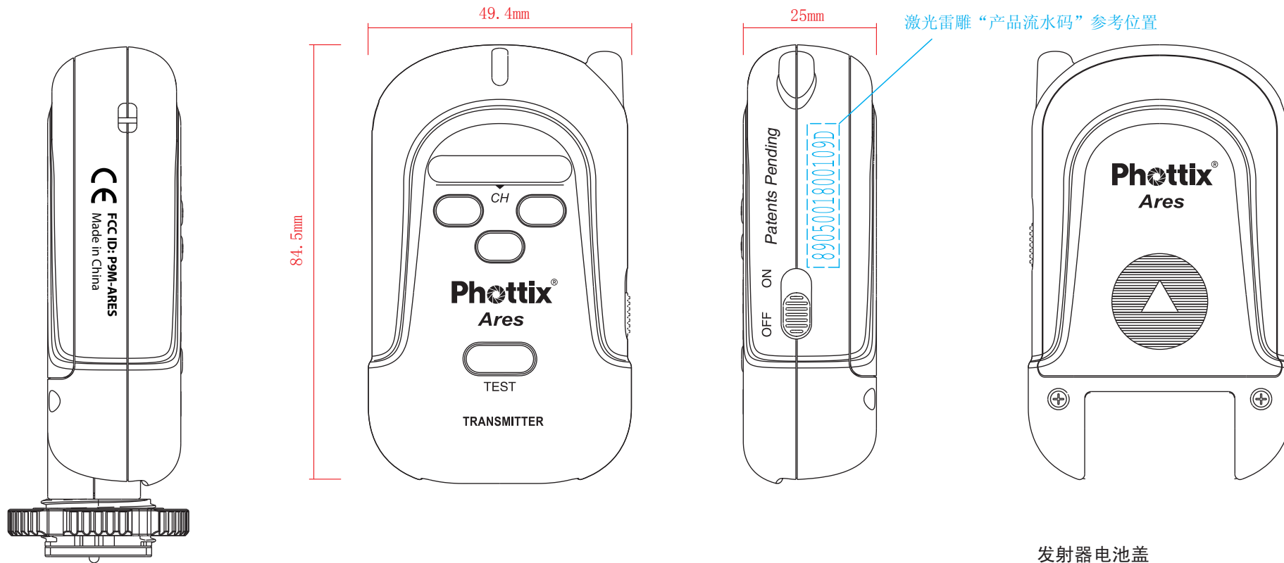
发射器上盖
