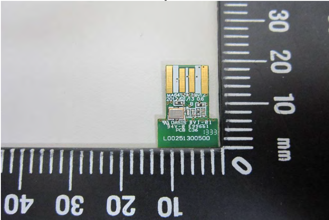
2.4GHz Antenna
