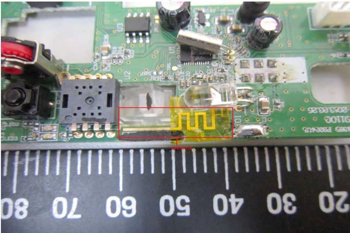
2.4GHz Antenna
