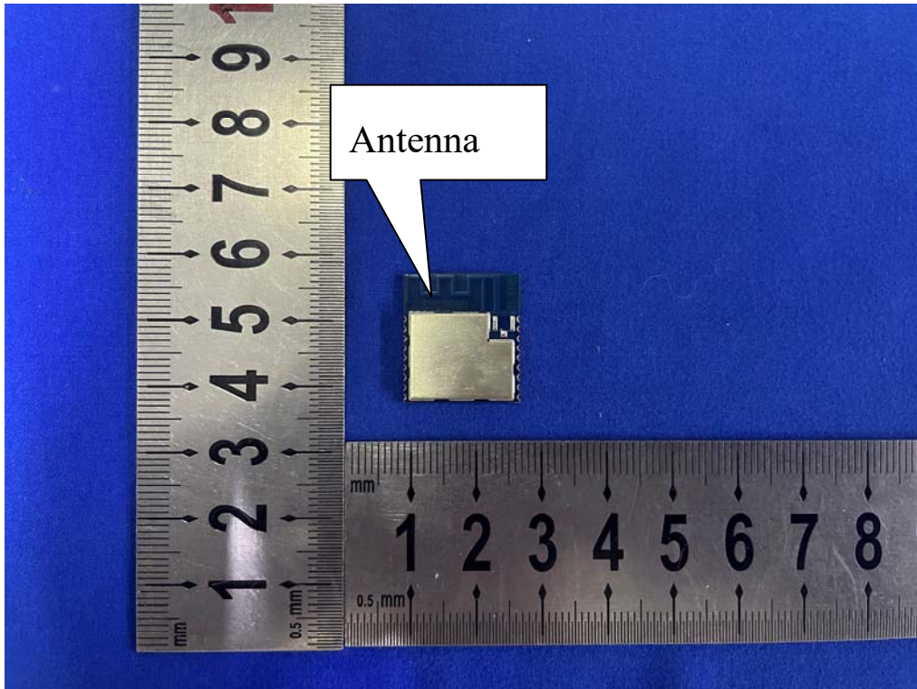
Photo 3:WIFI/BLE Antenna
