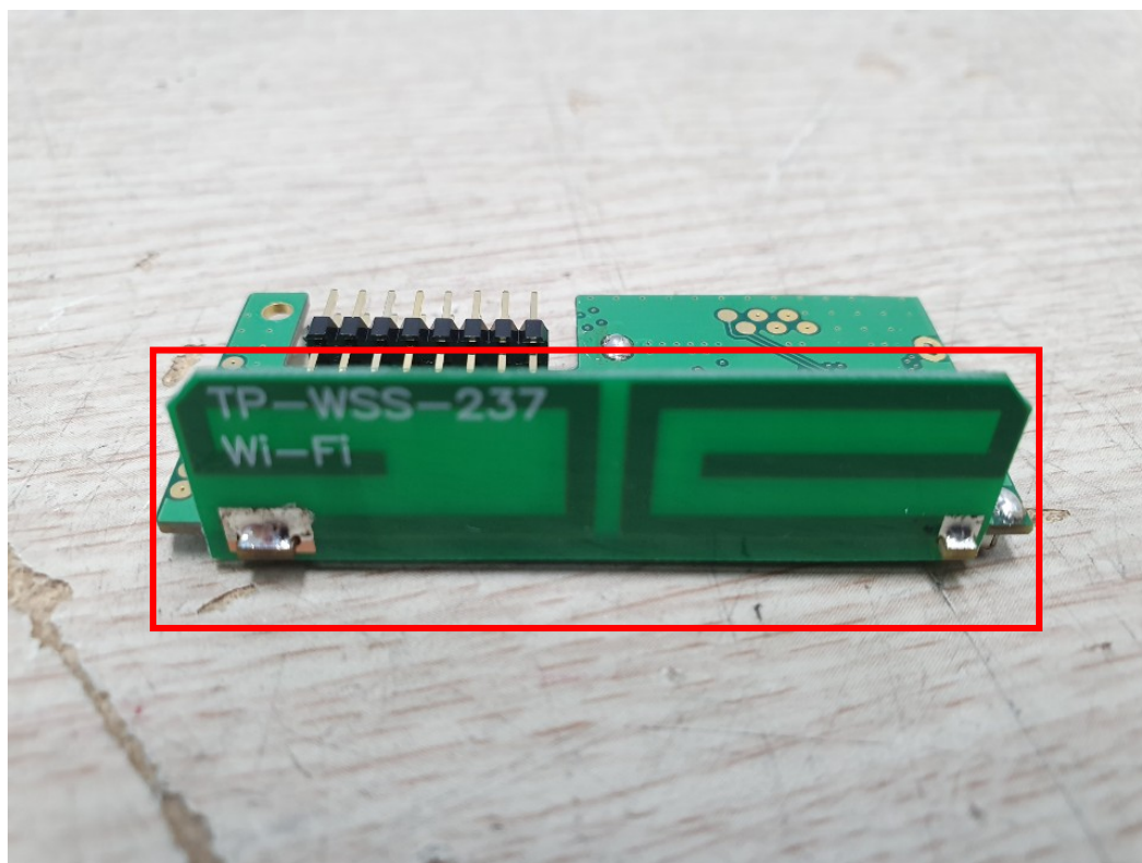
Antenna_WiFi 2.4 GHz
