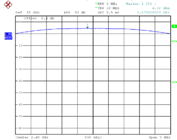
F6 (2 480 MHz)
