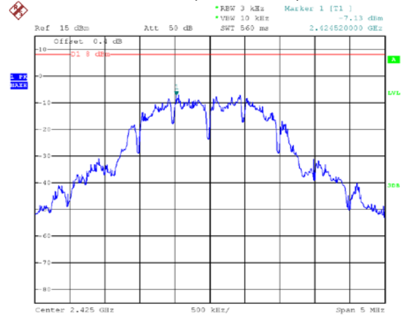
F2 (2 425 MHz)
