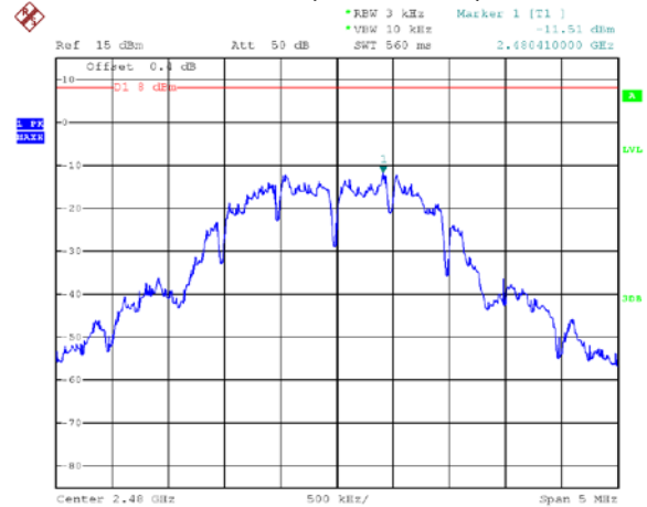
F6 (2 480 MHz)
