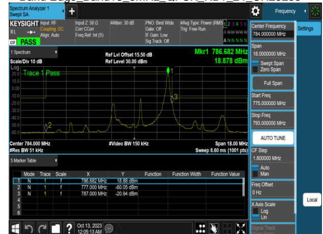
Band Edge_Band13_5MHz_QPSK_RB1_24_CH23255
