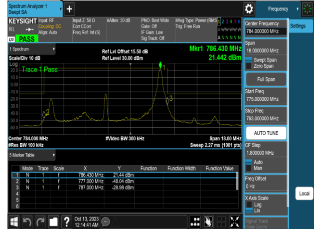
Band Edge_Band13_10MHz_QPSK_RB50_0_CH23230
