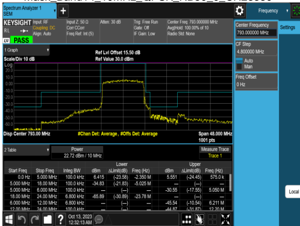
Mask_Band14_10MHz_QPSK_RB50_0_CH23330
