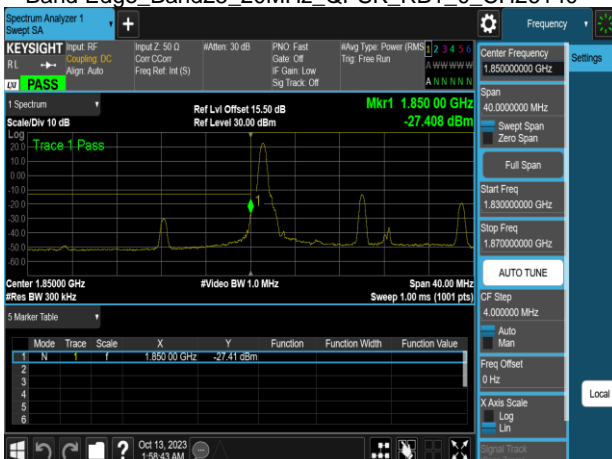
Band Edge_Band25_20MHz_QPSK_RB1_0_CH26140
