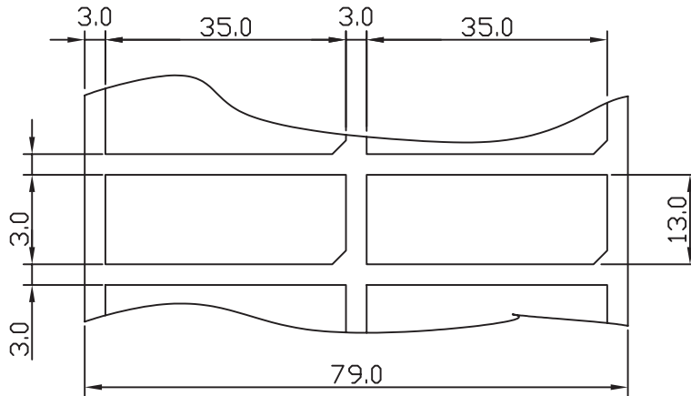
< 刀模圖 > 1:1
