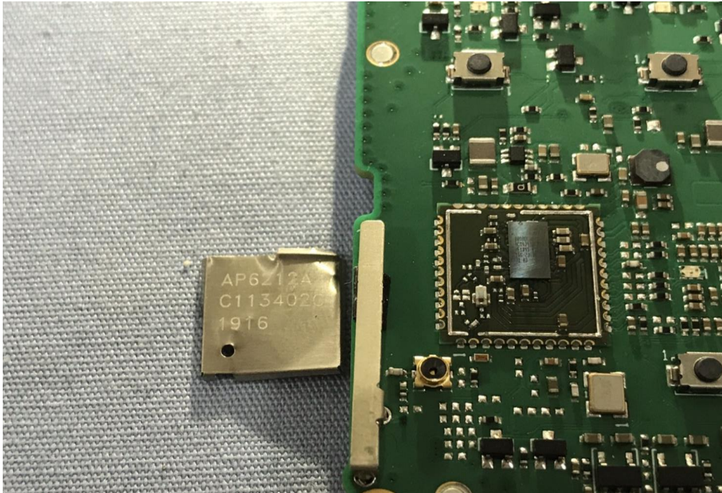
RF IC
