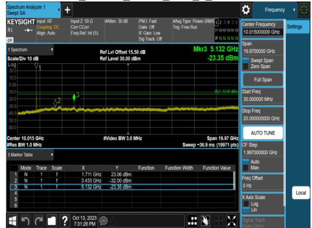
Band4_10MHz_QPSK_RB1_0_CH20175
