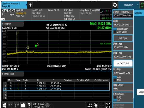
Band25_20MHz_QPSK_RB1_0_CH26590
