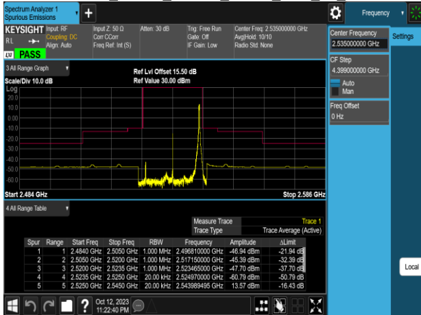
Emission Mask_Band7_20MHz_QPSK_RB1_99_CH21350
