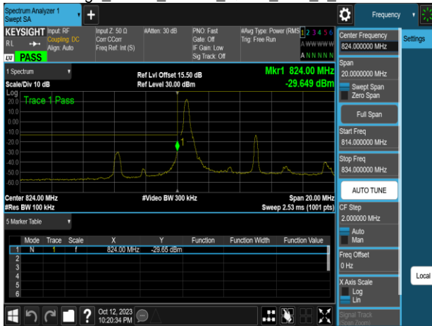
Band Edge_Band5_10MHz_QPSK_RB1_49_CH20600
