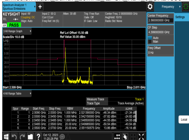
Emission Mask_Band7_20MHz_QPSK_RB1_0_CH21350
