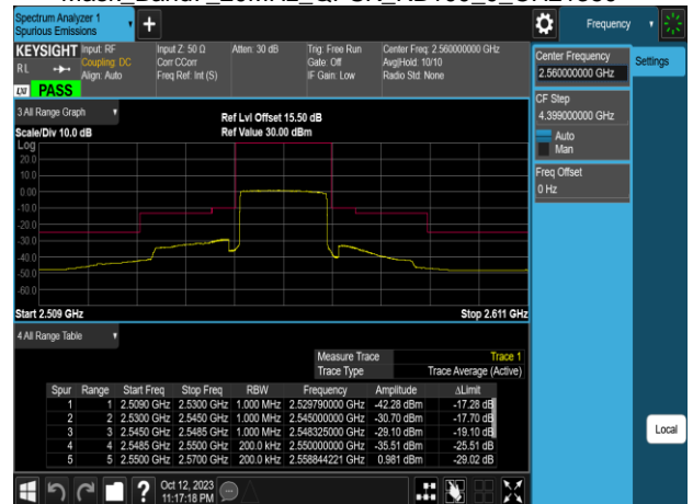
Emission Mask_Band7_20MHz_QPSK_RB100_0_CH21350
