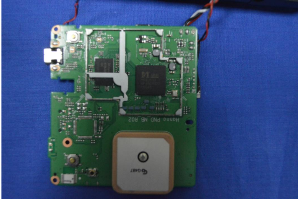
(5) EUT Photo
