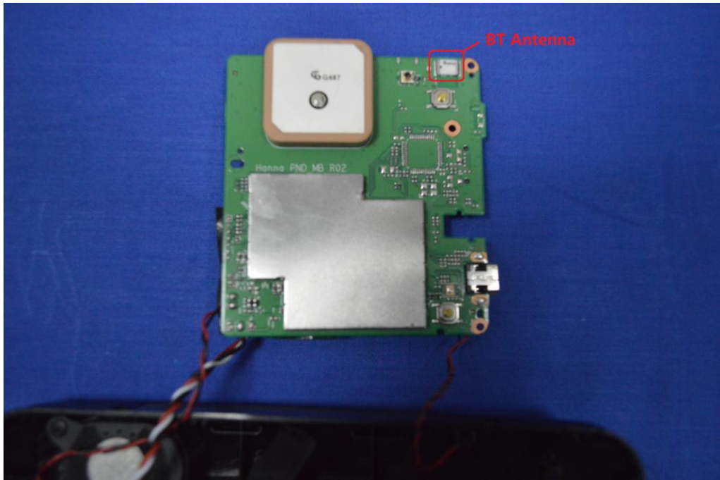
(4) EUT Photo
