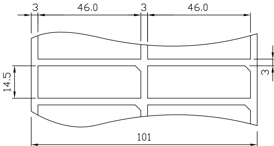
< 刀模圖 > 1:1
