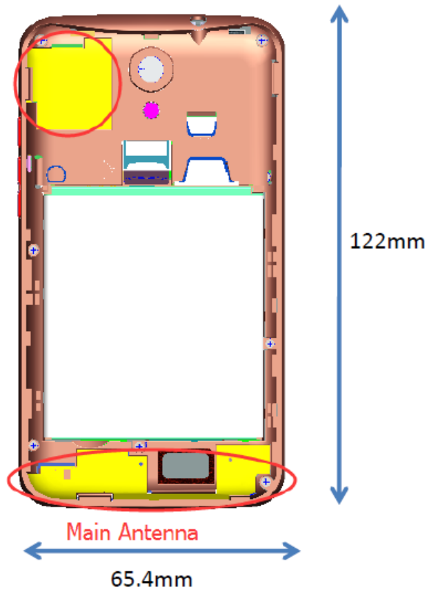
BT/WIFI/GPS Antenna
