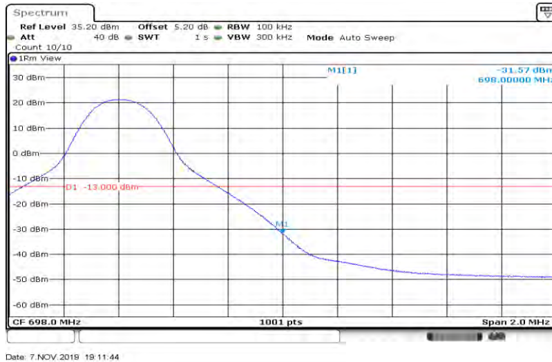
Band71-10MHz-QPSK-133422-50RB#0
