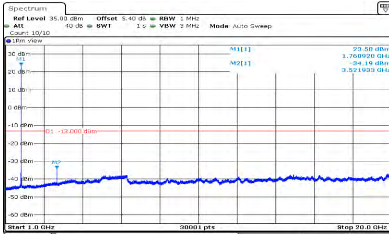
Band66-20MHz-QPSK-132572-1RB#0-Range2:1000~20000MHz
