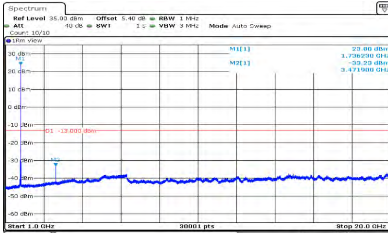
Band66-20MHz-QPSK-132322-1RB#0-Range2:1000~20000MHz
