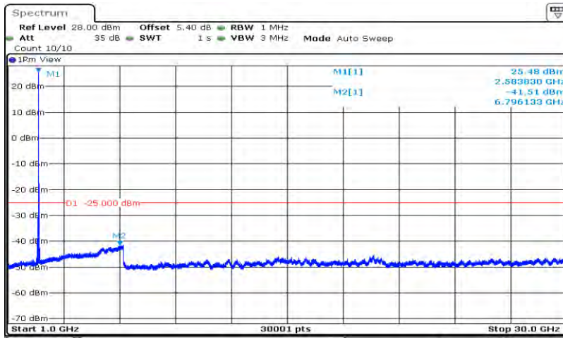
Band41-20MHz-QPSK-40620-1RB#0-Range2:1000~30000MHz
