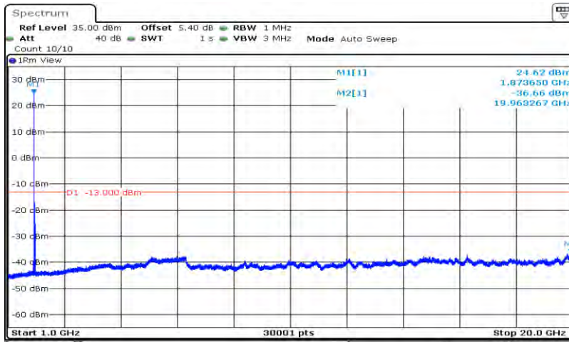
Band25-20MHz-16QAM-26365-1RB#0-Range2:1000~20000MHz
