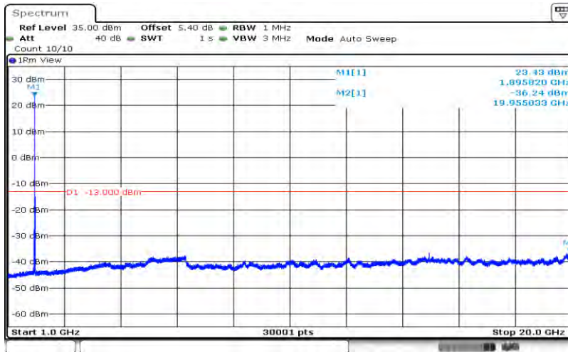
Band25-20MHz-QPSK-26590-1RB#0-Range2:1000~20000MHz
