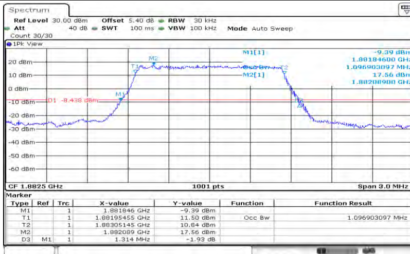
Band25-1.4MHz-QPSK-26365-6RB#0-1.097
