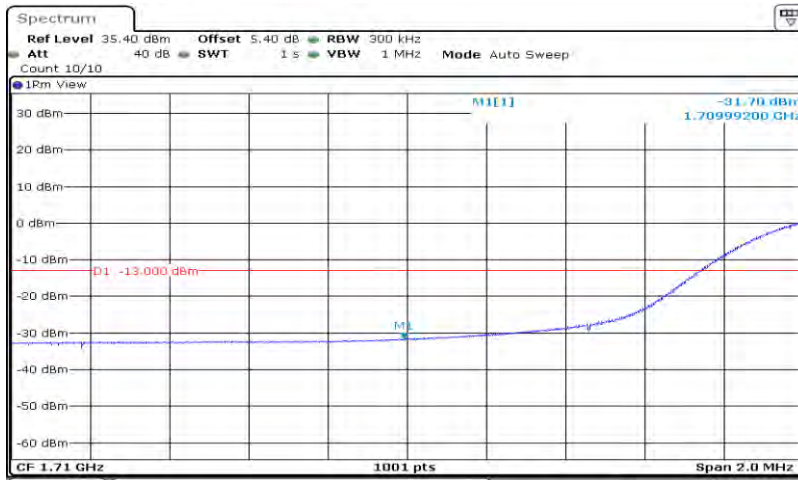
Band4-20MHz-QPSK-20050-100RB#0
