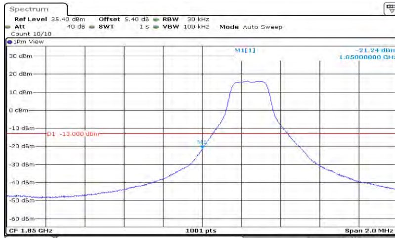
Band2-3MHz-16QAM-18615-15RB#0
