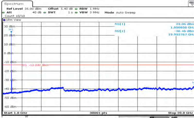
Band2-20MHz-16QAM-18700-1RB#0-Range2:1000~20000MHz
