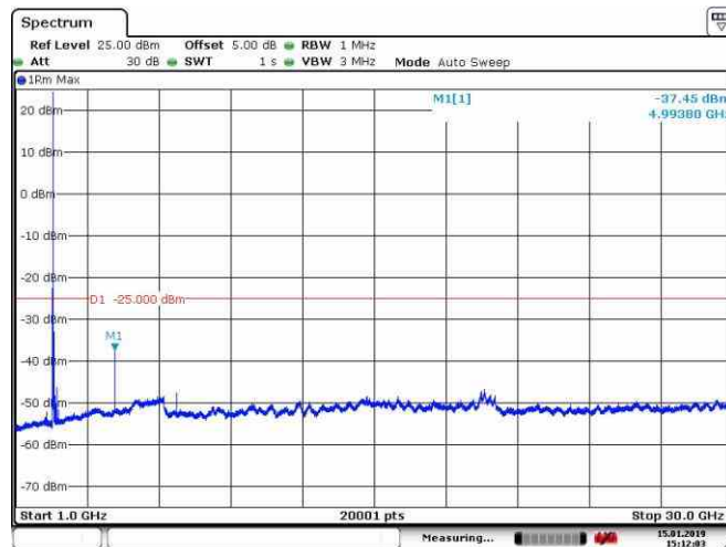
Band41_20MHz_QPSK_39750_1RB#0
