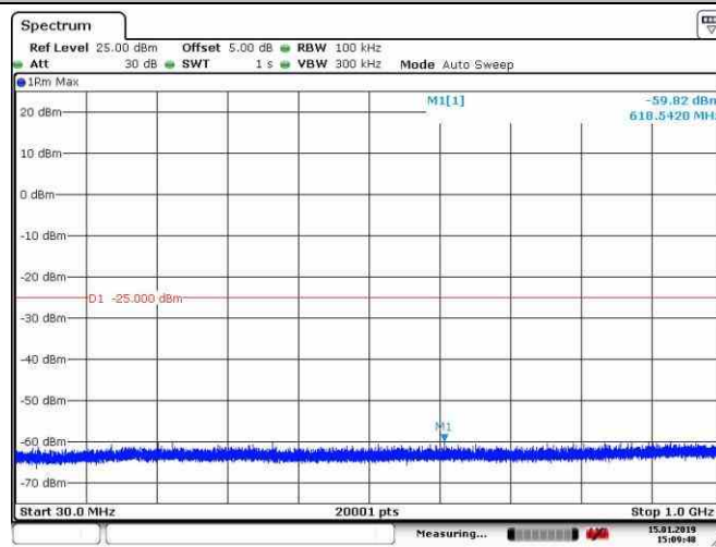
Band41_20MHz_QPSK_39750_1RB#0
