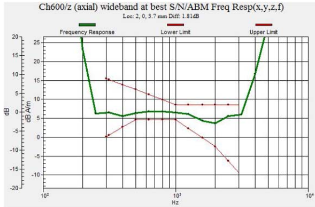
Fig. 9.5 CDMA2000 BC1 Ch600
