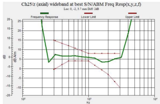
Fig. 9.4 CDMA2000 BC1 Ch25
