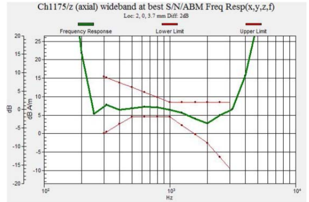
Fig. 9.6 CDMA2000 BC1 Ch1175
