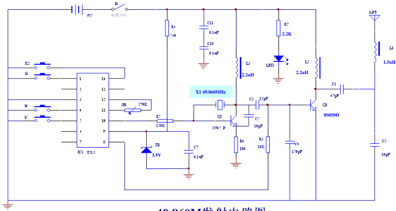
49.860M发射电路图
