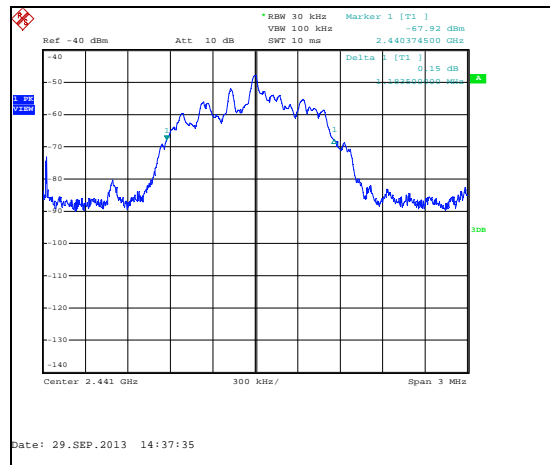
Figure 7.3.2-8: 20dB BW Mid CH ( \pi/4 DQPSK - 2Mbps)
