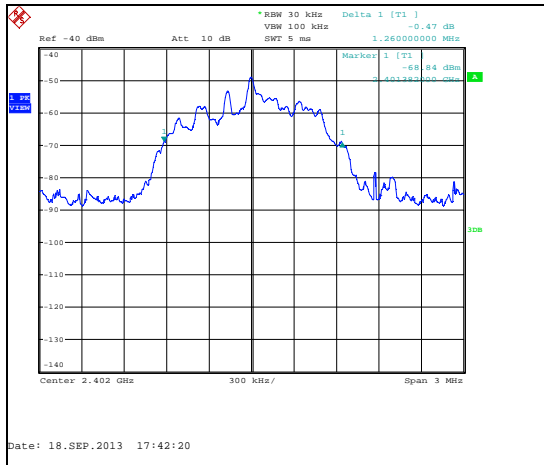
Figure 7.3.2-7: 20dB BW Low CH ( \pi/4 DQPSK - 2Mbps)
