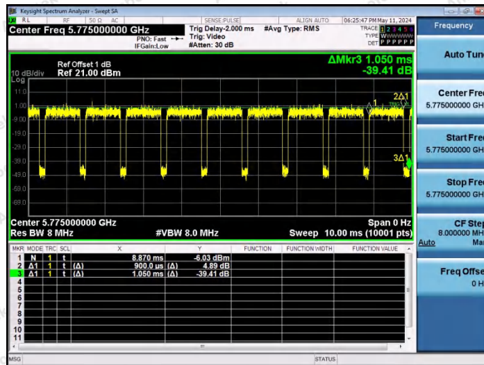
NTNV-11AC80SISO-Ant1-5775
