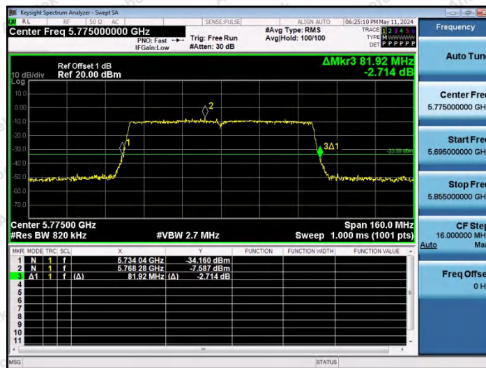
11AC80SISO-Ant1-5775
