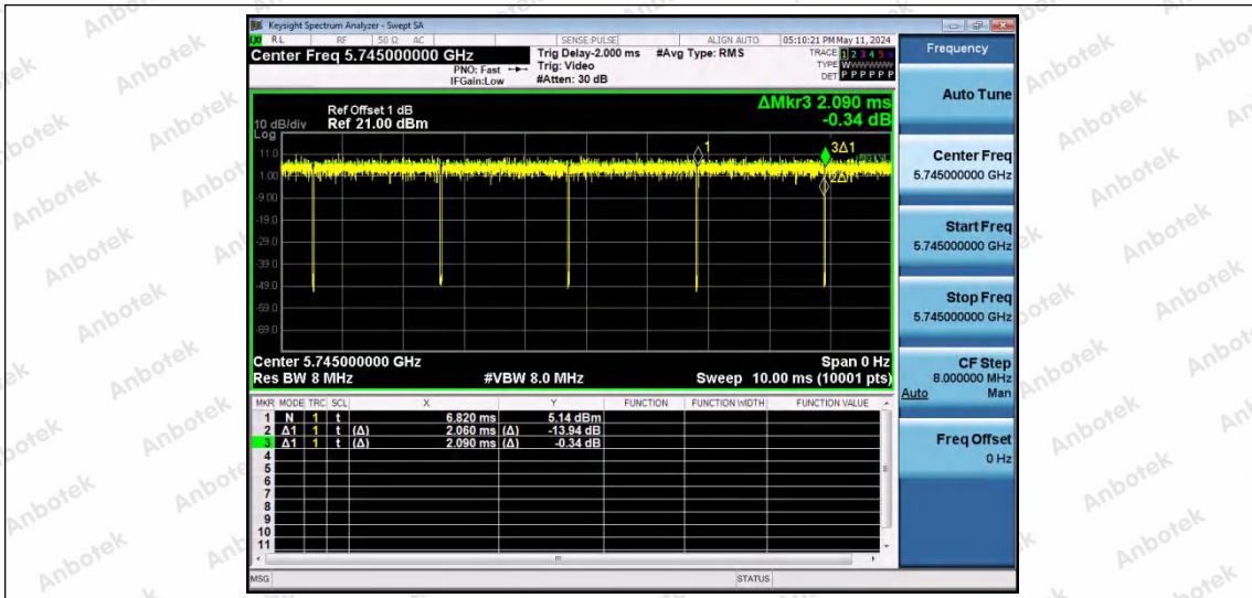
NTNV-11A-Ant1-5745
