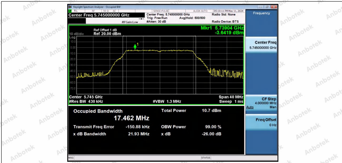
11A-Ant1-5745
