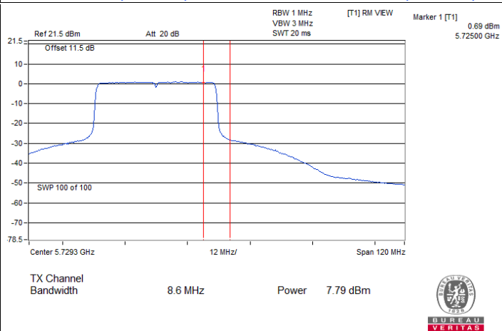
802.11be (EHT40) CDD / Chain 1 : CH 142 (U-NII-3)
