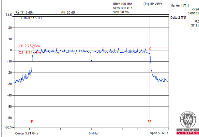
802.11be (EHT40) / Chain 2 : CH 142 (U-NII-3)
