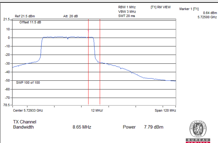
802.11be (EHT40) CDD / Chain 0 : CH 142 (U-NII-3)
