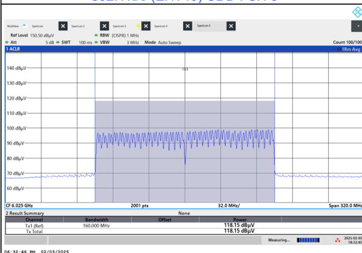
802.11be (EHT160) CDD : CH 15
