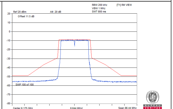
802.11be (EHT20) / Chain 3 : CH 45
