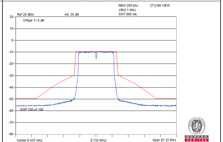
802.11be (EHT20) / Chain 3 : CH 97
