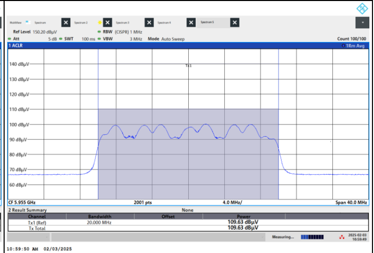
802.11be (EHT20) CDD : CH 1
