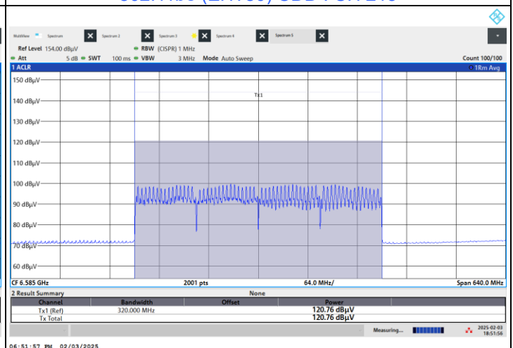
802.11be (EHT320) CDD : CH 127
