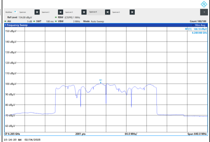
802.11be (EHT320) Beamforming : CH 63
