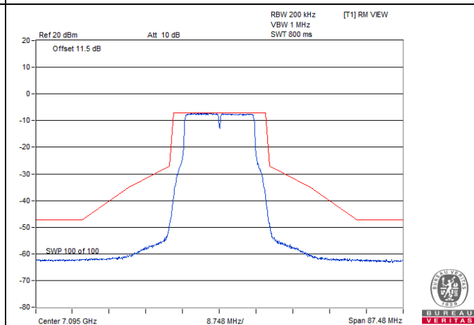
802.11a / Chain 3 : CH 229
