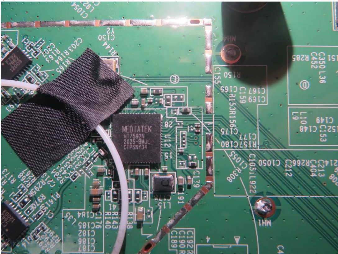
(10) EUT Photo
