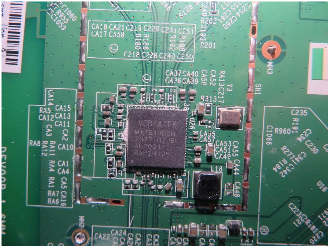
(12) EUT Photo
