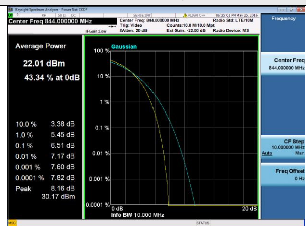
10MHz / 64QAM
