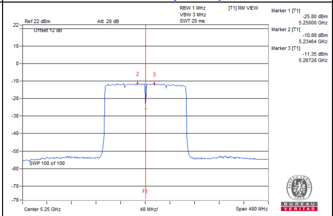
802.11ax (HE160)
