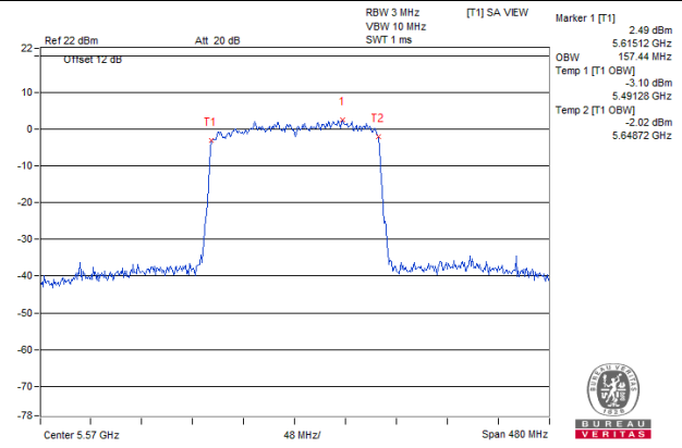
802.11ax (HE160)
