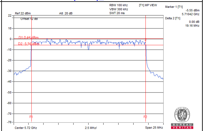
802.11ax (HE20)_Chain 3: CH 144
