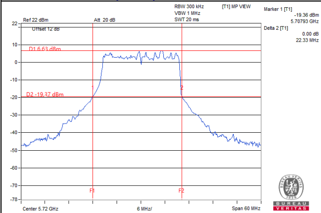
802.11ax (HE20) _Chain 2: CH 144
