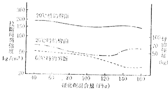
圖 II 2.1 硬化劑混合量と粘り強度 (在20°C七天的硬化) 試驗片：軟銅板 (25×100×1.6mm) (Over-lap)12.5mm
