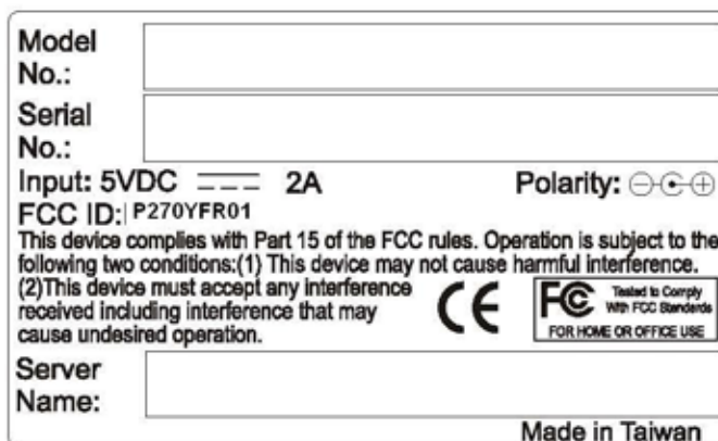
SCALE 2:1
