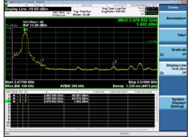
2480MHz(2.4GHz – 2.5GHz)
