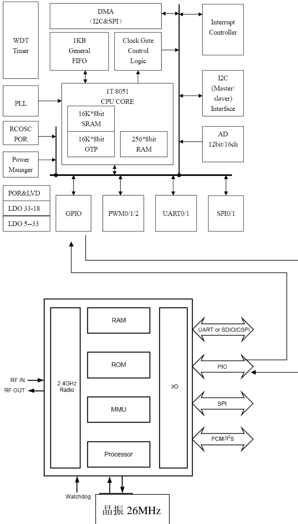
MARB0201 方框图
