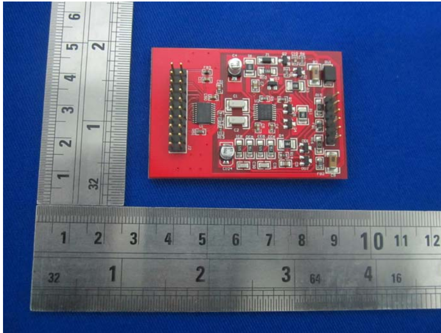
UT – FXO Board Bottom View
