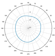
Total_Polar_H_5.85GHz
