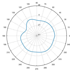
Total_Polar_E1_5.85GHz
