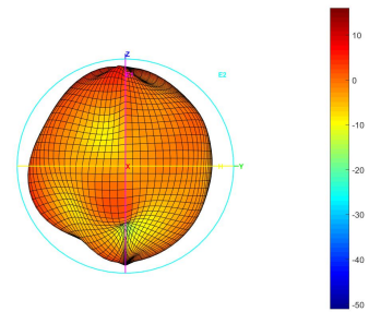
Total_3D_E2_5.85GHz
