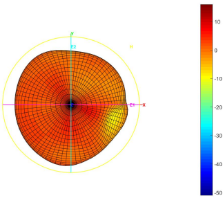
Total_3D_H_5.85GHz
