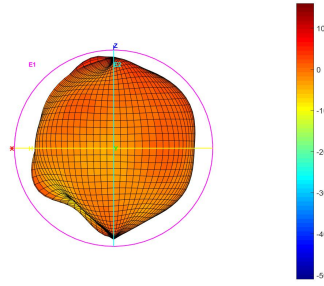
Total_3D_E1_5.85GHz
