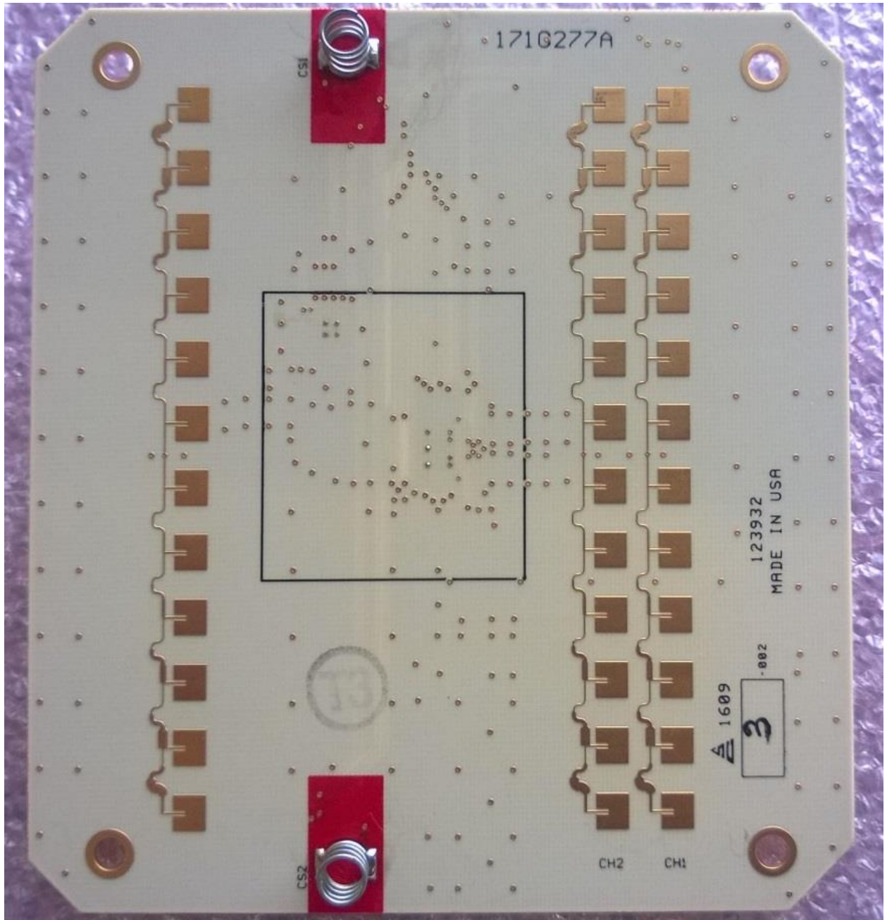
Antenna PCA Front
