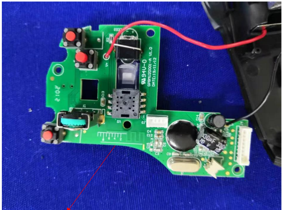
2.4G Antenna
