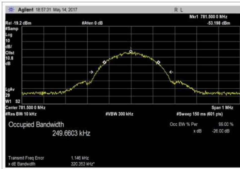
Input_OBW_UL_776-787MHz_GSM
