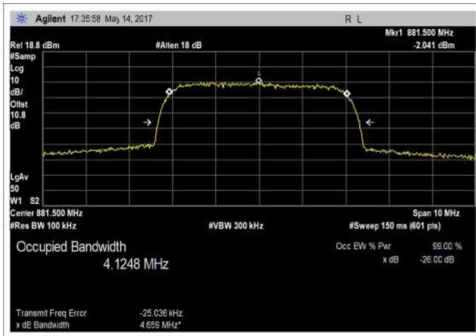
Output_OBW_DL_869-894MHz_WCDMA
