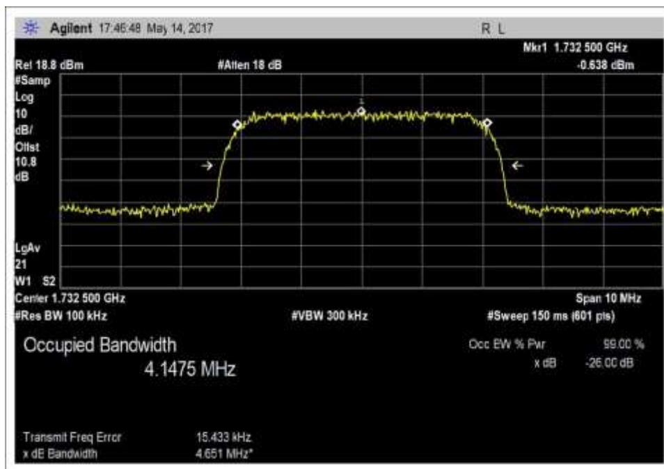
Output_OBW_UL_1710-1755MHz_WCDMA
