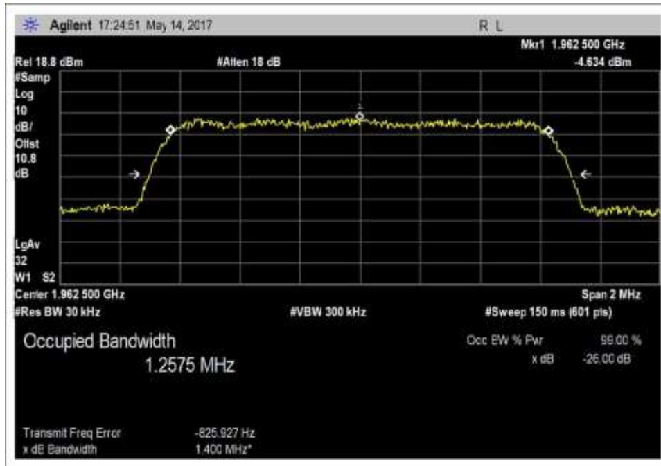
Output_OBW_DL_1930-1995MHz_CDMA
