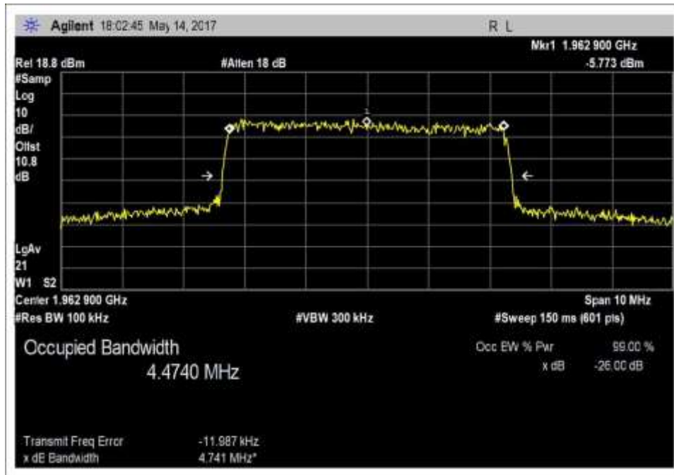
Output_OBW_DL_1930-1995MHz_LTE
