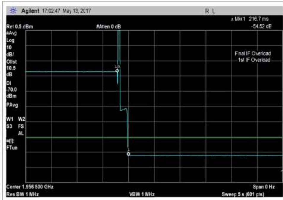
DL-1930-1995MHz
