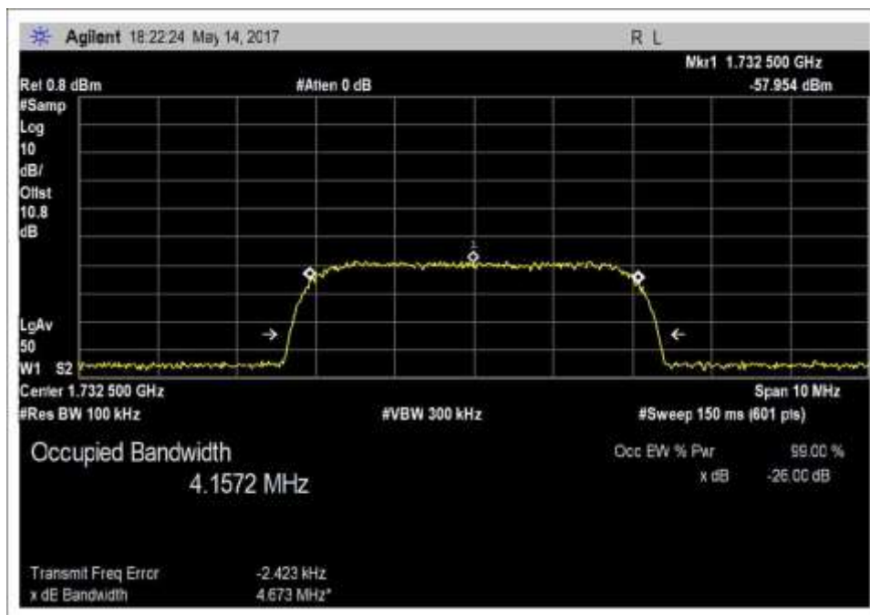
Input_OBW_UL_1710-1755MHz_WCDMA
