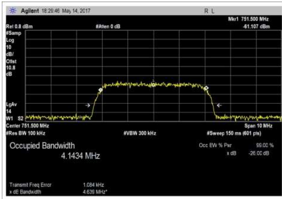
Input_OBW_DL_746-757MHz_WCDMA
