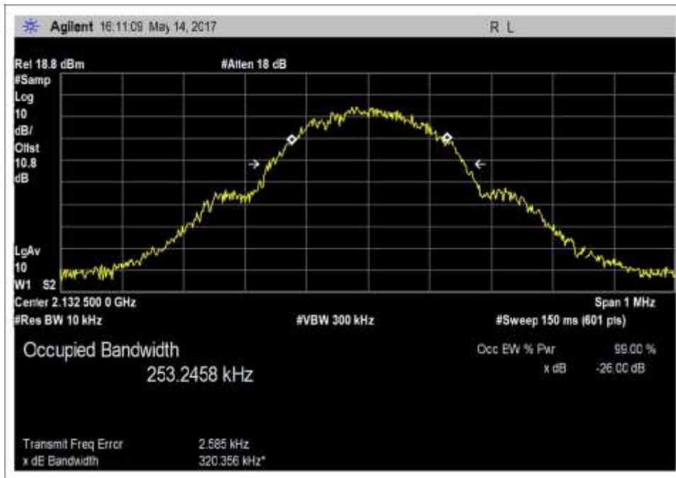
Output_OBW_DL_2110-2155MHz_GSM
