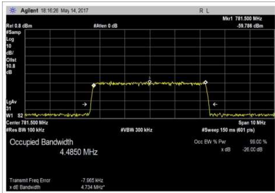
Input_OBW_UL_776-787MHz_LTE
