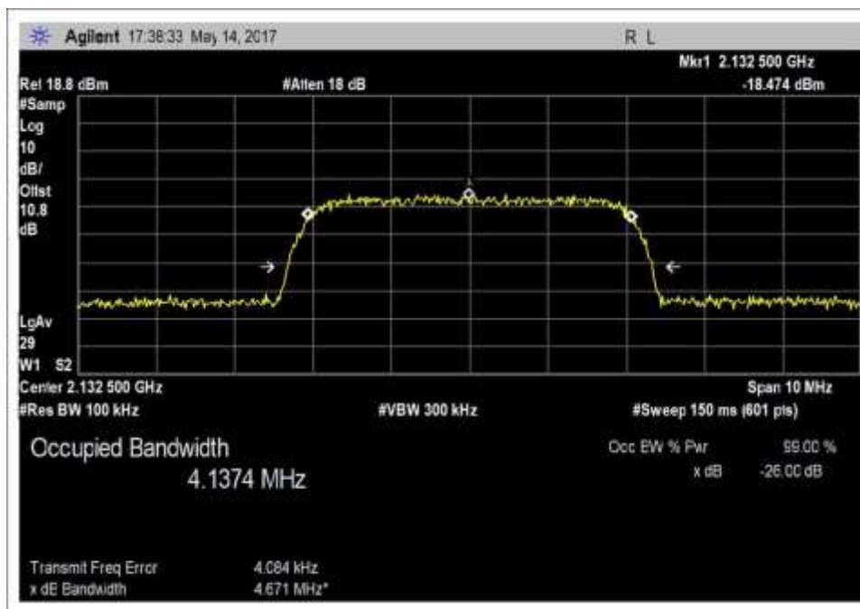
Output_OBW_DL_2110-2155MHz_WCDMA
