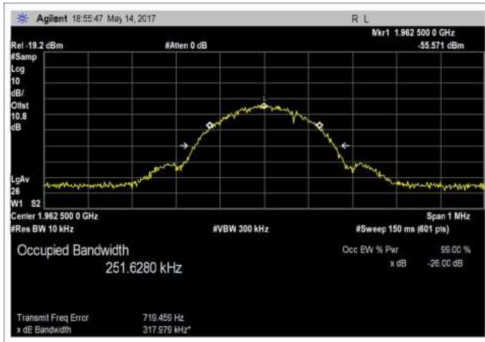
Input_OBW_DL_1930-1995MHz_GSM
