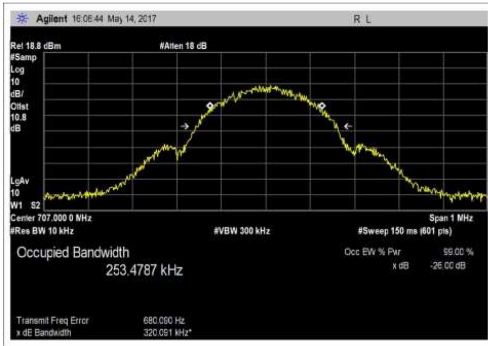
Output__OBW_UL_698-716MHz_GSM
