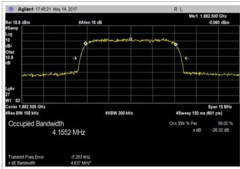
Output_OBW_UL_1850-1915MHz_WCDMA
