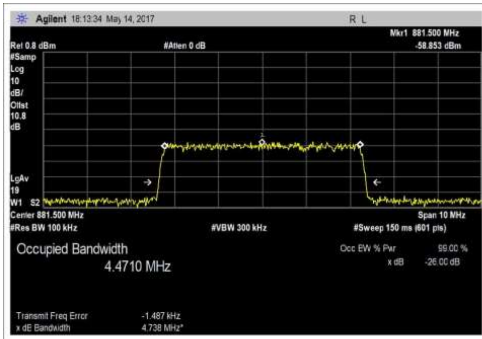
Input_OBW_DL_869-894MHz_LTE
