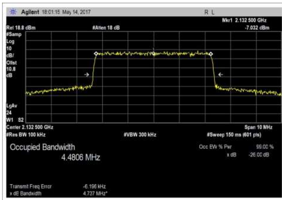
Output_OBW_DL_2110-2155MHz_LTE
