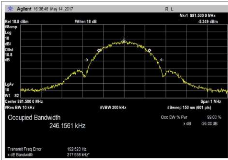
Output__OBW_DL_869-894MHz_EDGE
