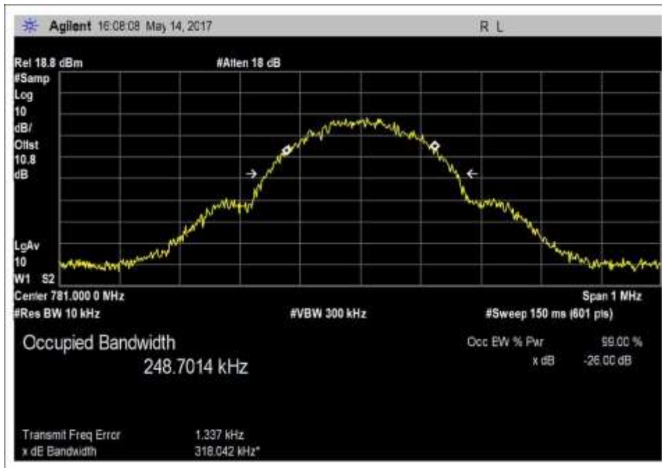
Output__OBW_UL 776-787MHz_GSM
