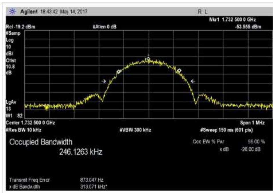
Input_OBW_UL_1710-1755MHz_EDGE
