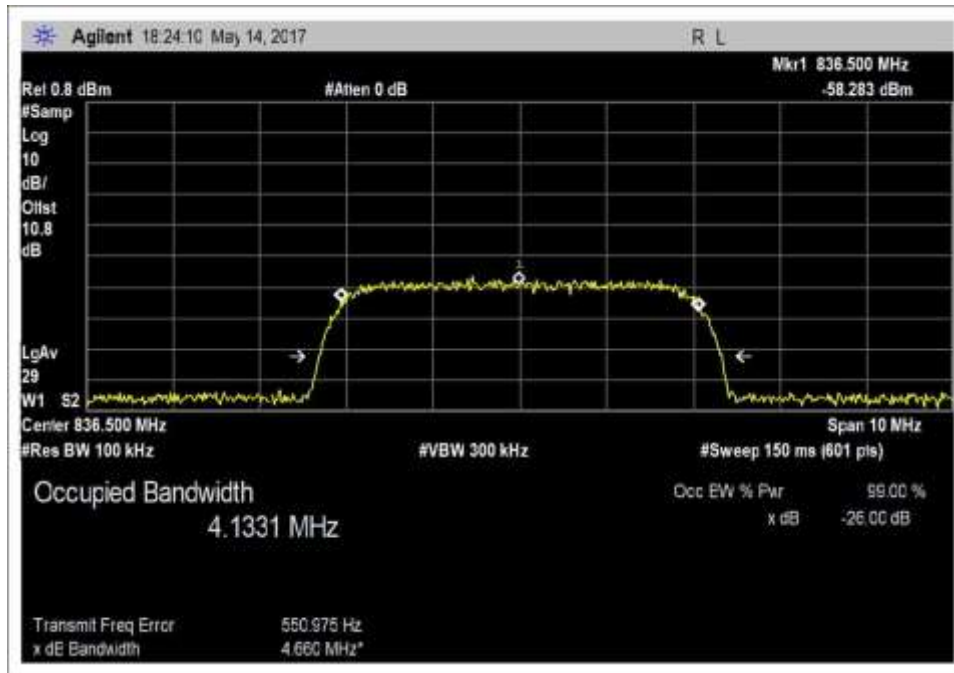
Input__OBW_UL_824-849MHz_WCDMA
