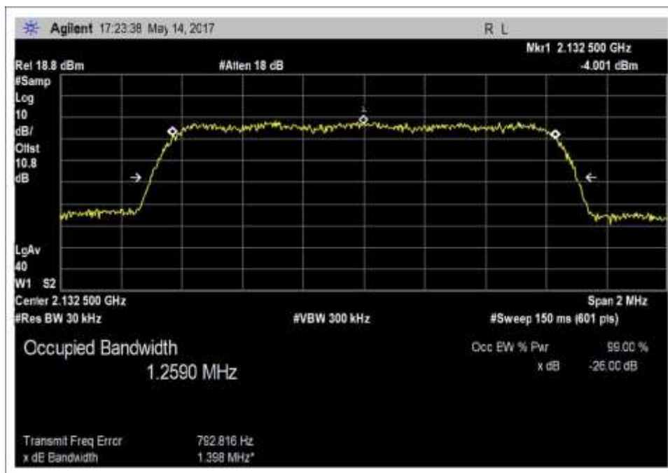
Output_OBW_DL_2110-2155MHz_CDMA
