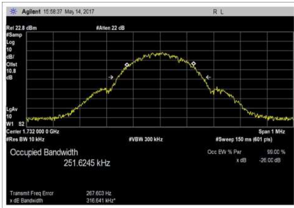
Output_OBW_UL_1710-1755MHz_GSM
