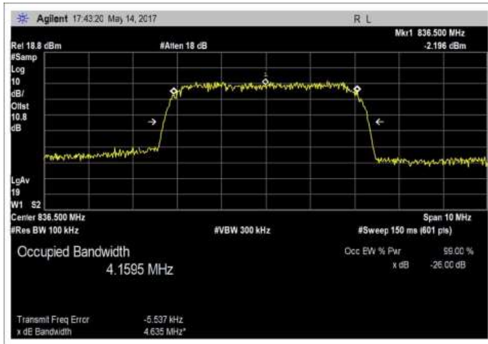
Output_OBW_UL_824-849MHz_WCDMA
