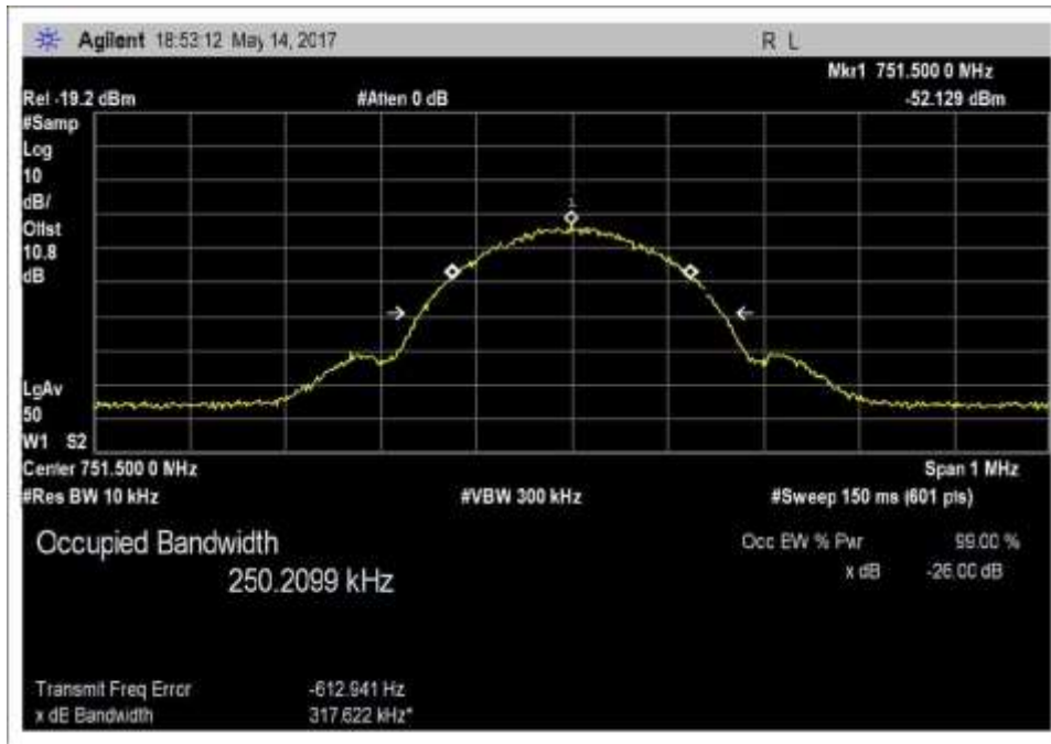
Input_OBW_DL_746-757MHz_GSM
