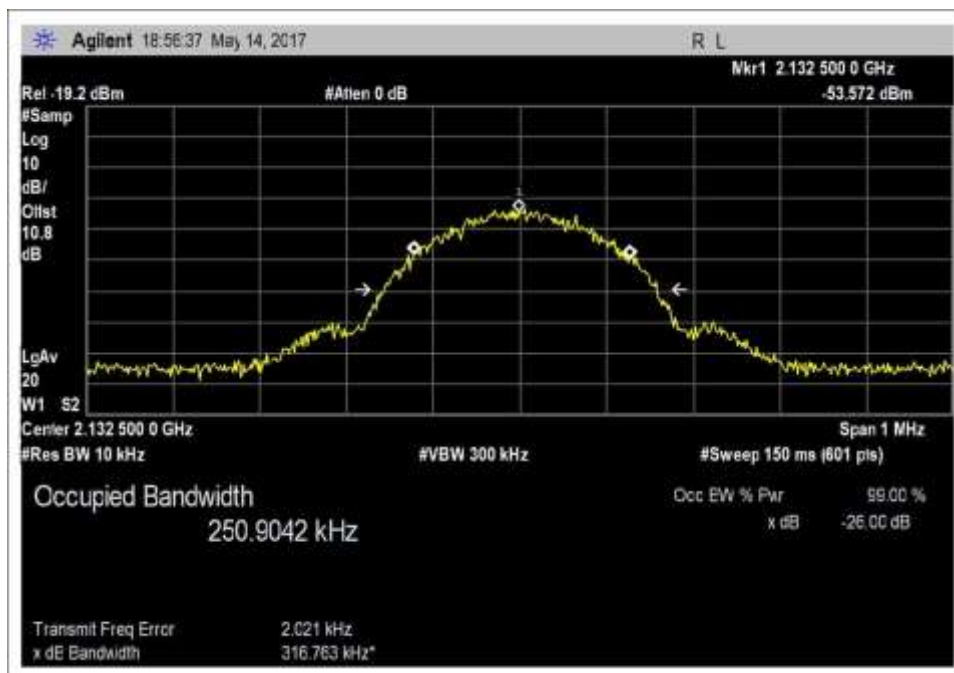
Input_OBW_DL_2110-2155MHz_GSM
