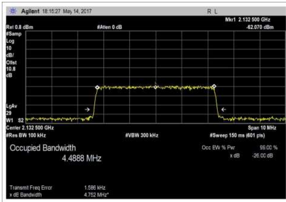
Input_OBW_DL_2110-2155MHz_LTE
