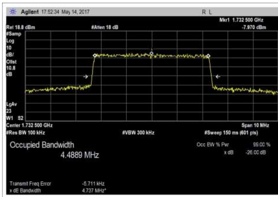
Output_OBW_UL_1710-1755MHz_LTE
