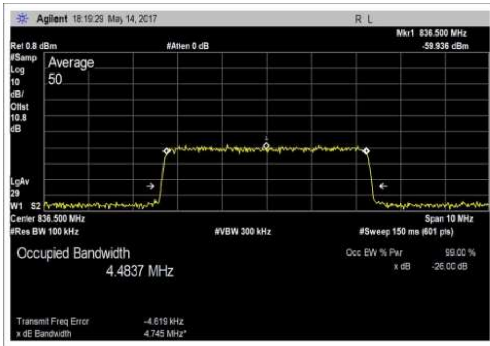
Input_OBW_UL_824-849MHz_LTE
