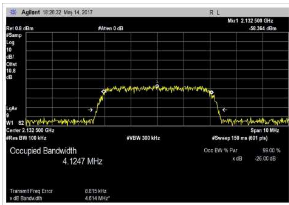
Input_OBW_DL_2110-2155MHz_WCDMA
