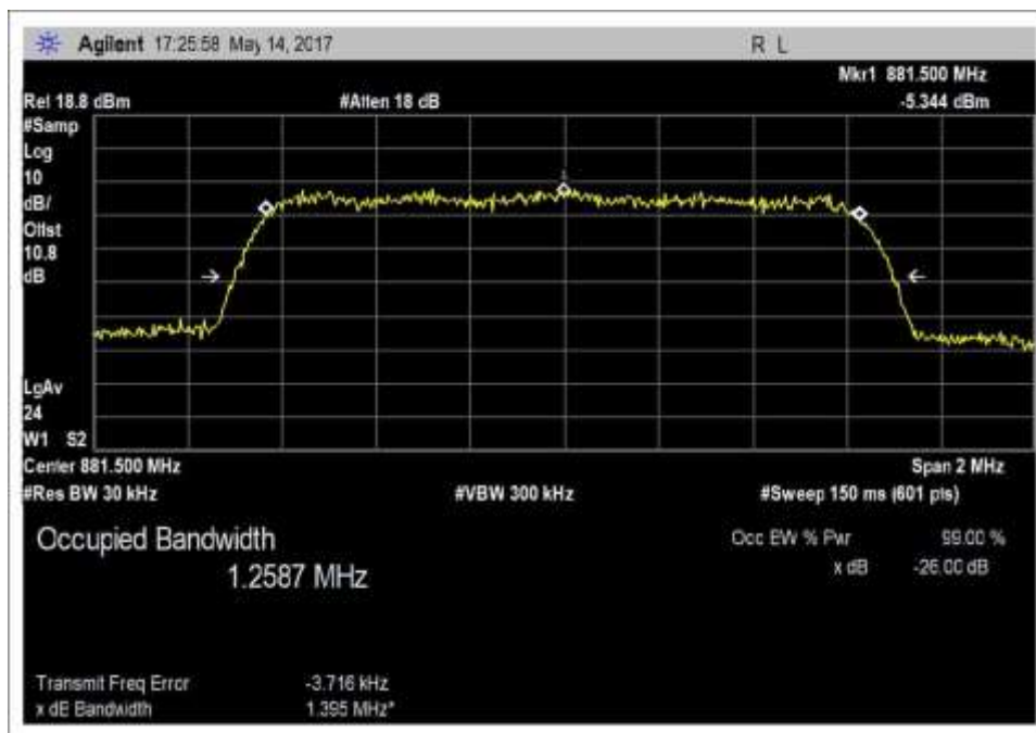
Output_OBW_DL_869-894MHz_CDMA
