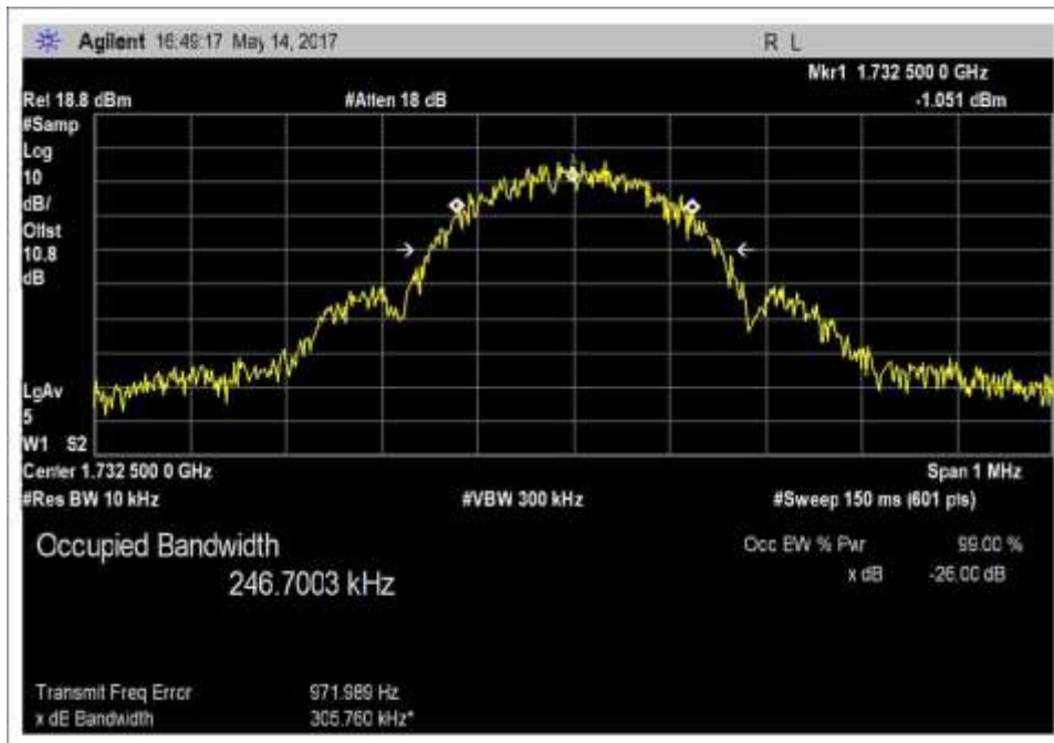
Output_OBW_UL_1710-1755MHz_EDGE
