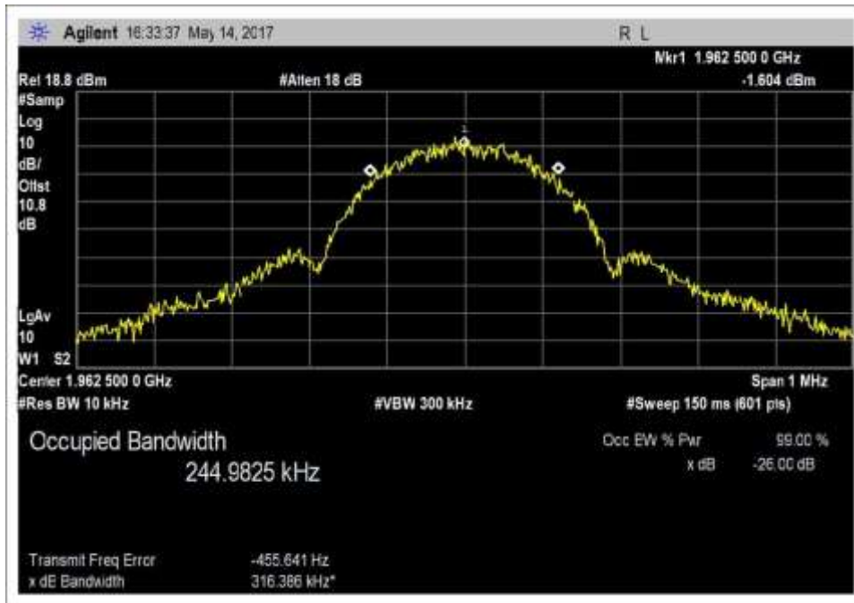
Output_OBW_DL_1930-1995MHz_EDGE
