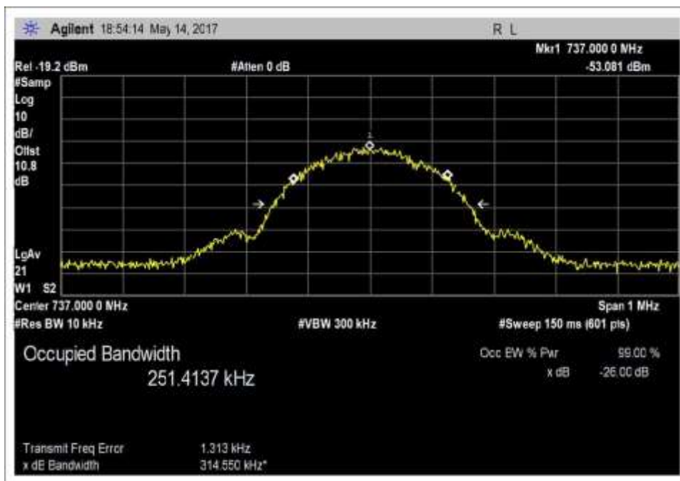
Input_OBW_DL_728-746MHz_GSM
