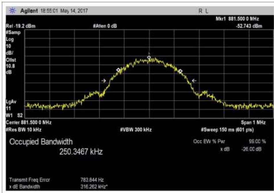
Input_OBW_DL_869-894MHz_GSM
