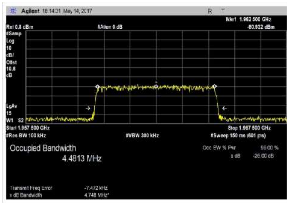
Input_OBW_DL_1930-1995MHz_LTE
