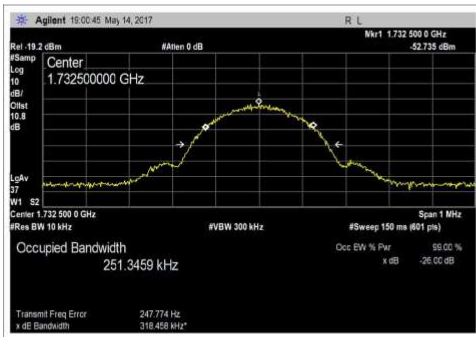
Input_OBW_UL_1710-1755MHz_GSM
