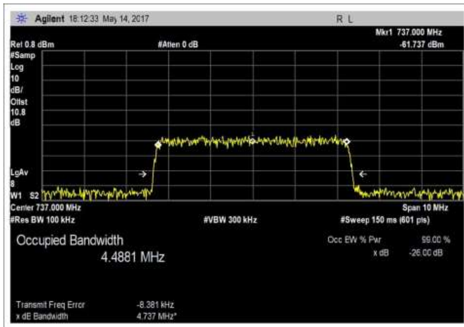
Input_OBW_DL_728-746MHz _LTE
