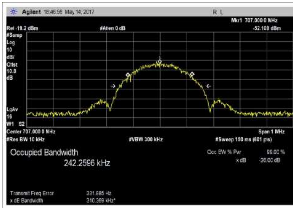
Input_OBW_UL_698-716MHz_EDGE
