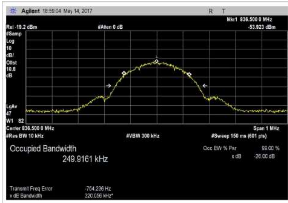
Input_OBW_UL_824-849MHz_GSM
