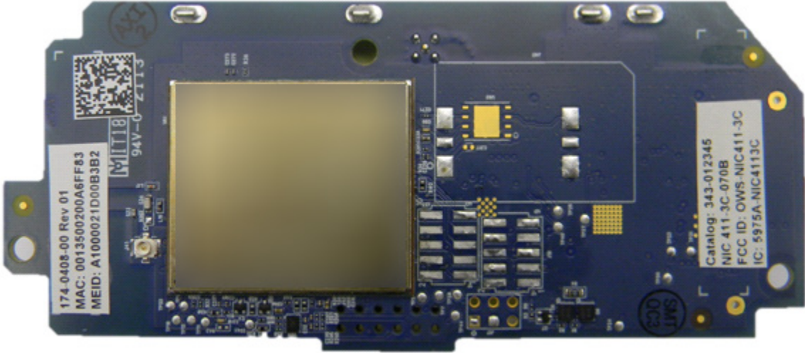
Bottom Side
