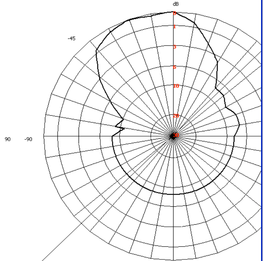
Site nb: 1008 - Vertical pattern
