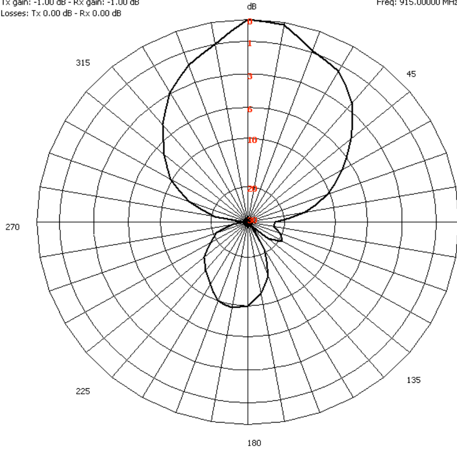
Site nb: 1008 - Horizontal pattern
